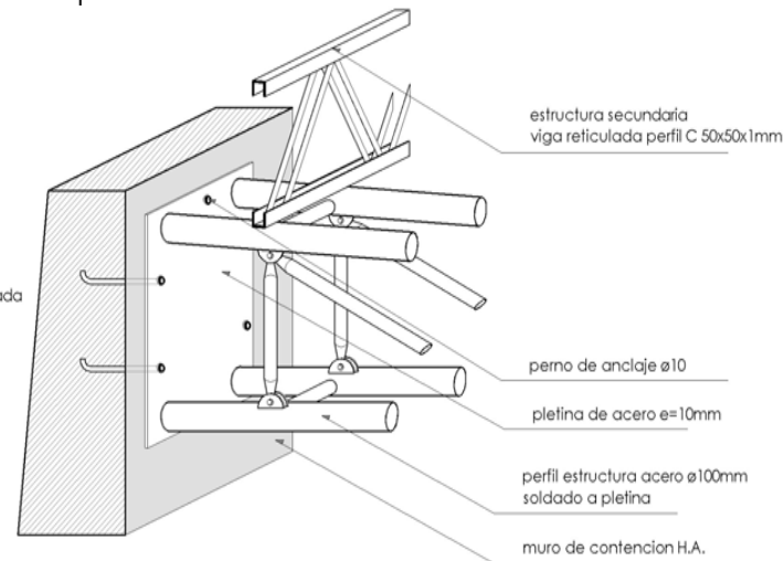
DETALLE TIPO unión viga muro
