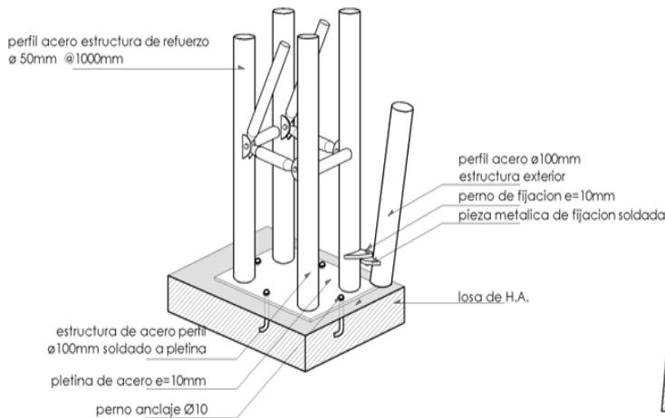
DETALLE TIPO unión pilar losa
