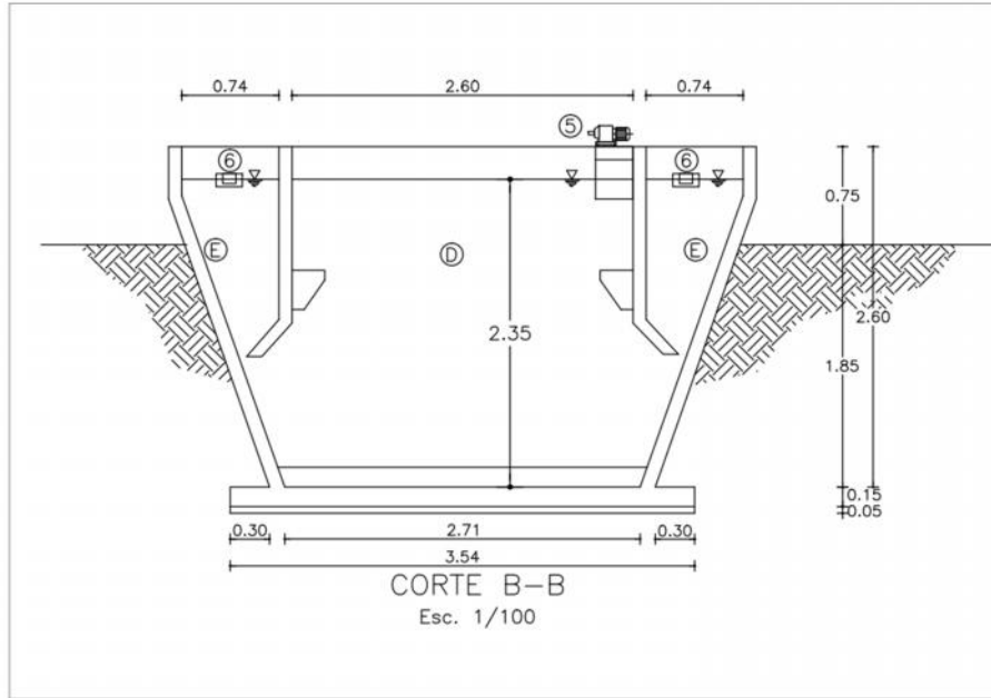
FIGURA 12. Corte B-B
