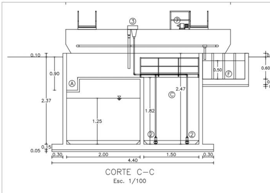
FIGURA 13. Corte C-C
