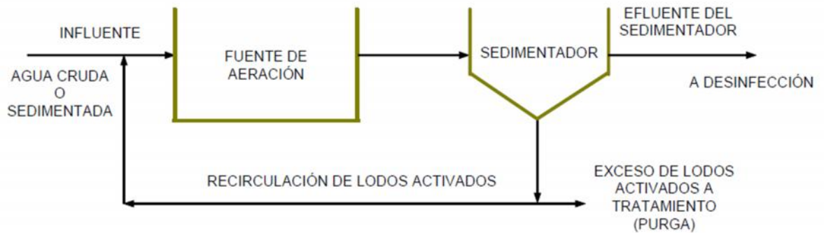
FIGURA 9. Proceso básico de lodos activados
