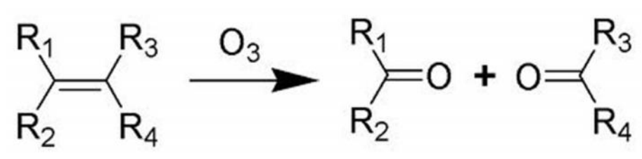
FIGURA 6. Reacción del ozono y formación de ozónidos
